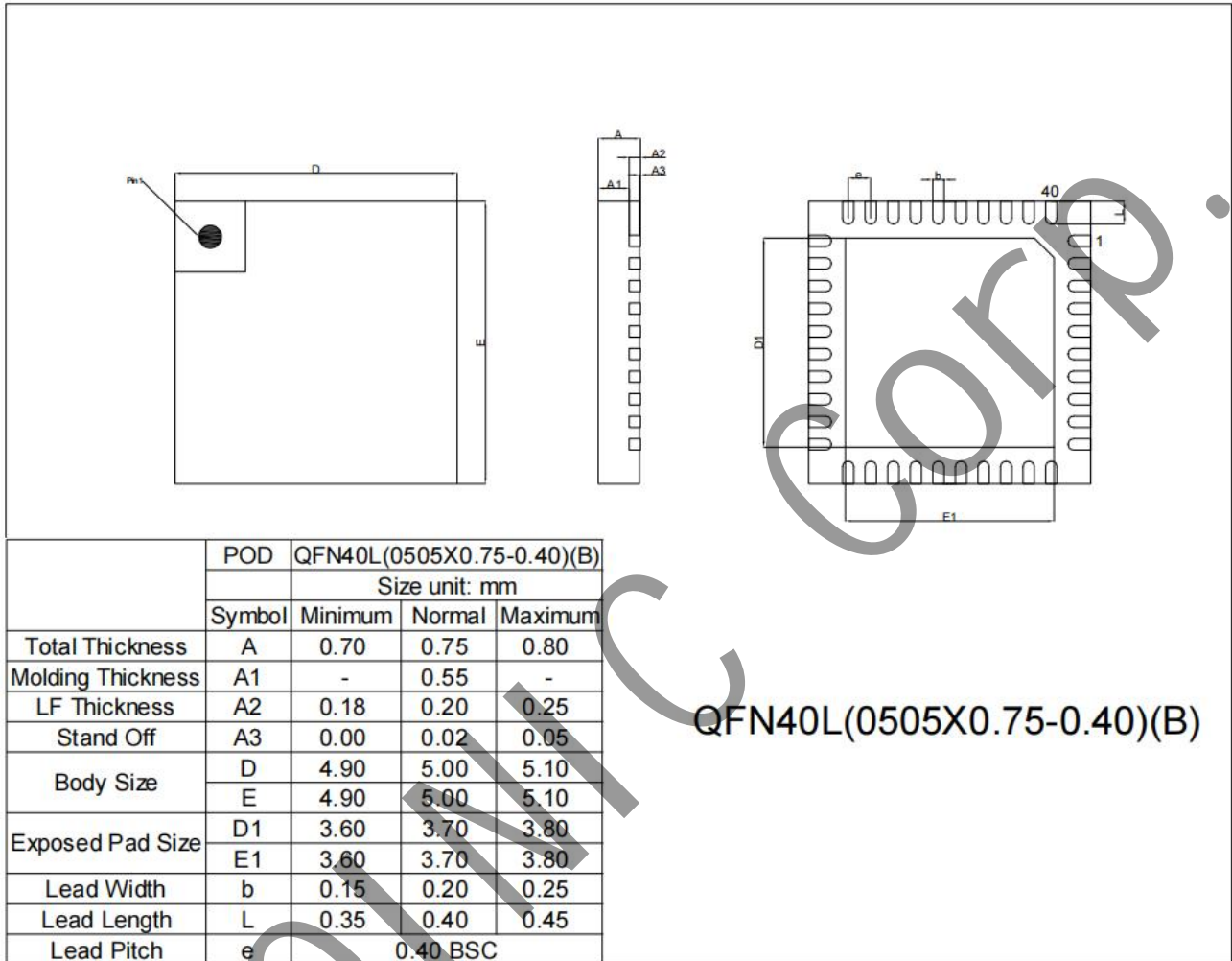
图 13 封装图
